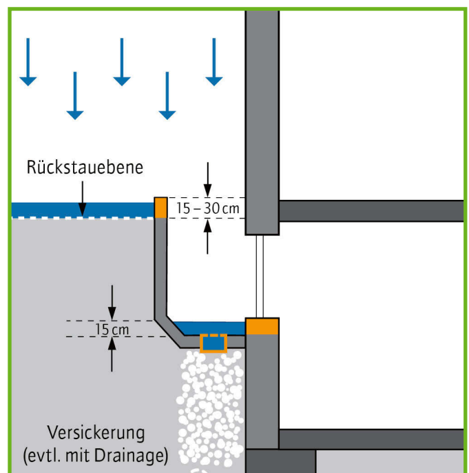
22b Lichtschacht | RICHTIG
