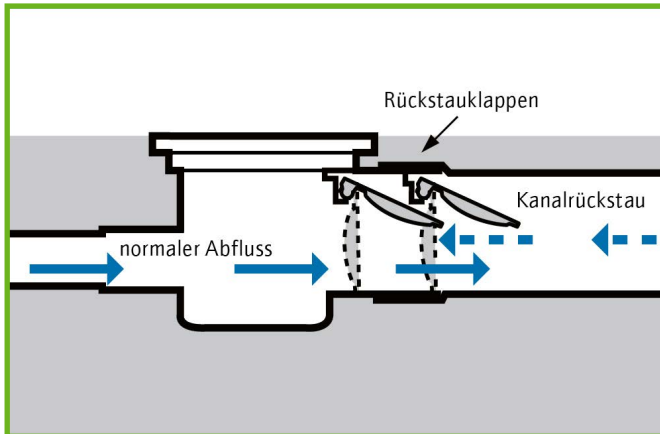
39 Funktionsweise einer Rückstauklappe
