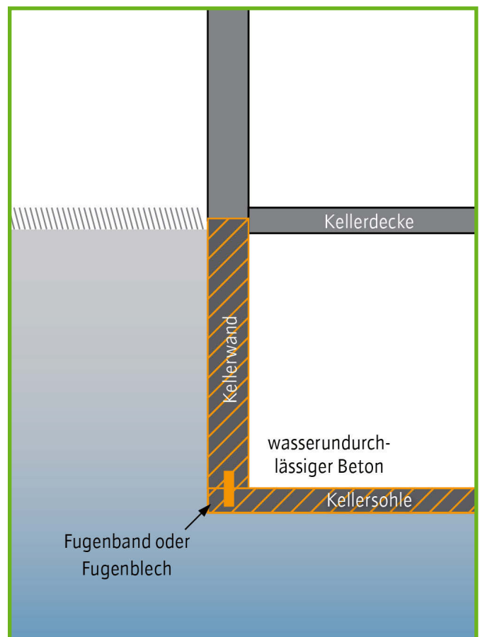
51b Weiße Wanne
