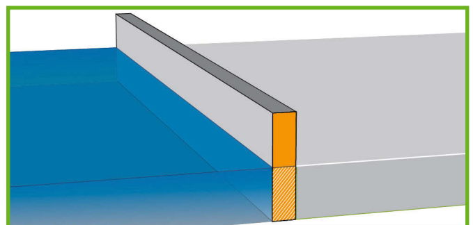
17 Unterirdische Abdichtung einer Schutzmauer
