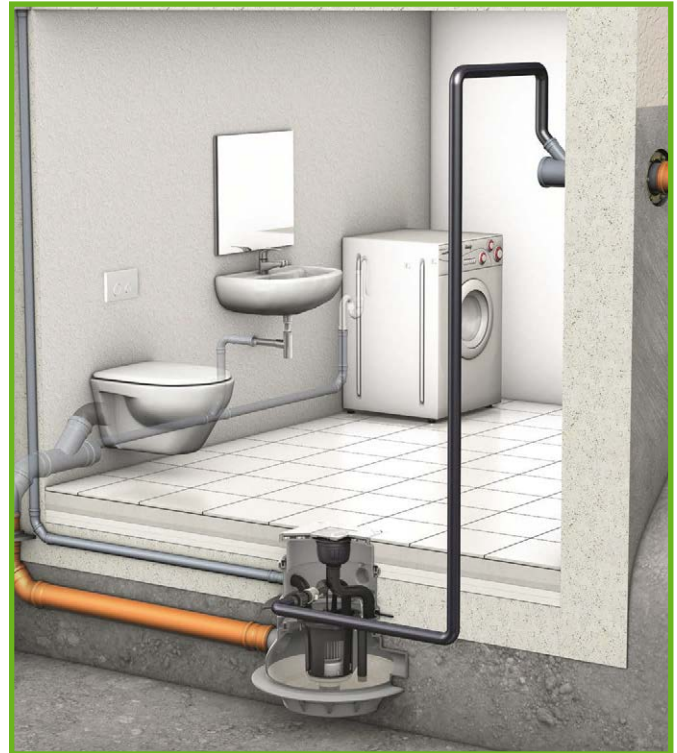
43 Funktionsprinzip einer Hebeanlage
