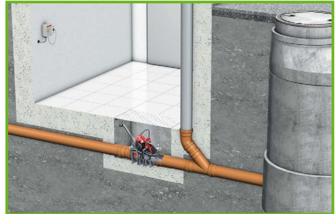
40 Funktionsweise einer Rückstauklappe
