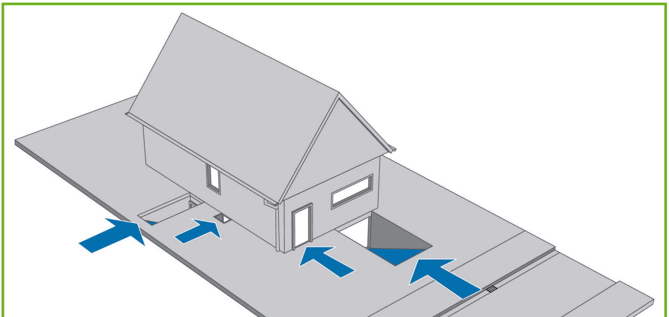
8 Eintrittswege für Starkregenabflüsse
