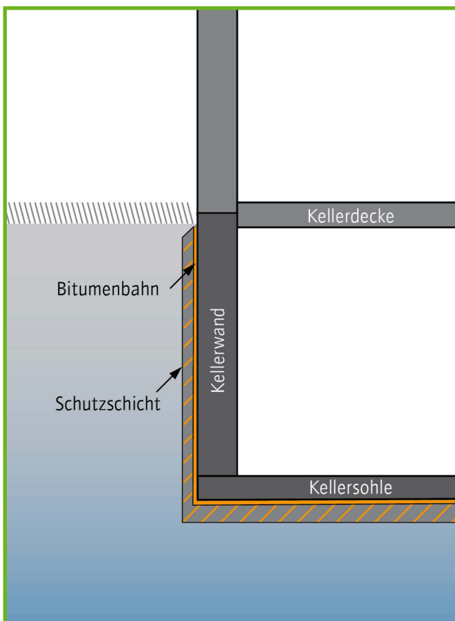
51a Schwarze Wanne
