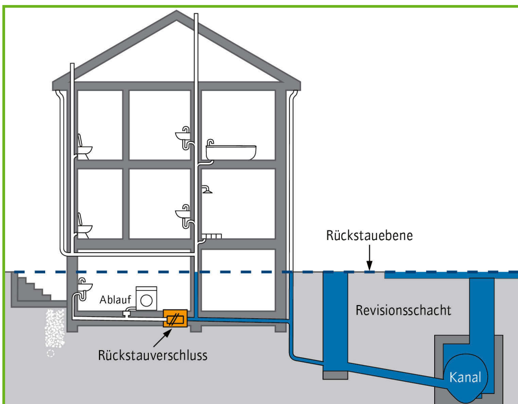
38a Rückstauverschluss | RICHTIG
