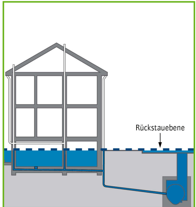
36 Rückstauebene
