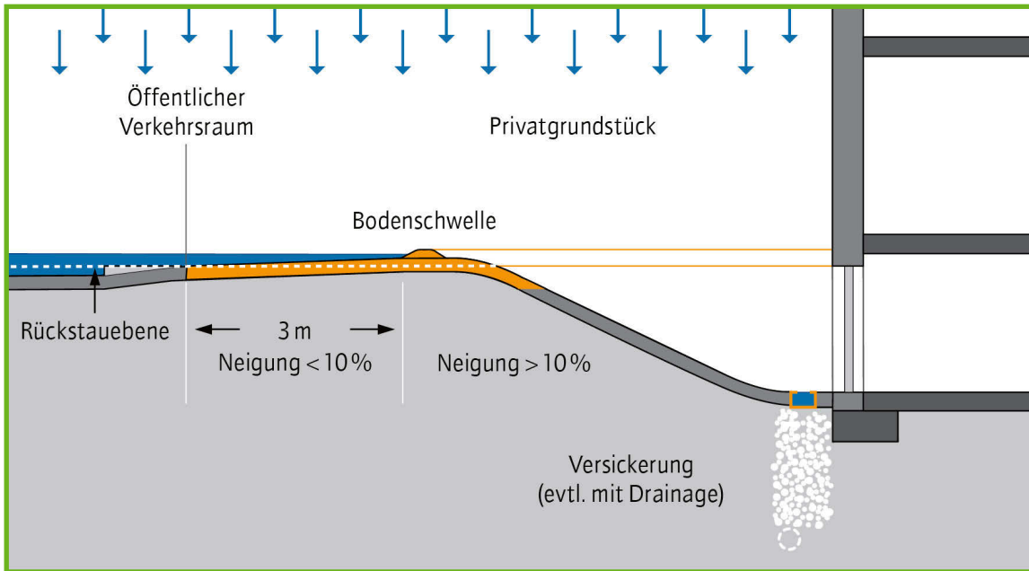
18 Bodenschwelle vor Tiefgarazufahrt
