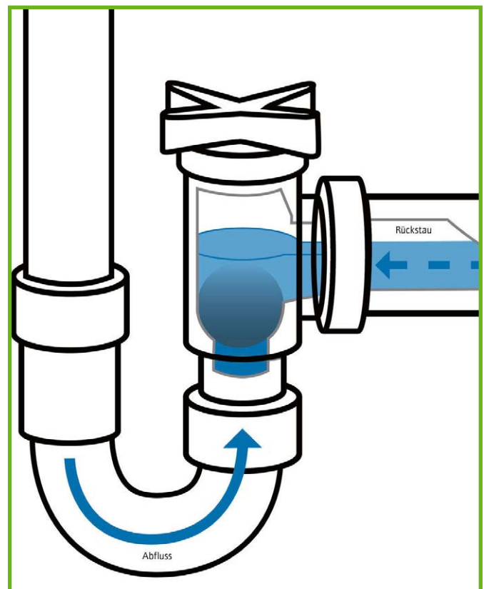
45 Siphon mit Kugelschluss
