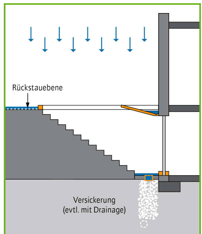
19b Kellertreppe | RICHTIG
